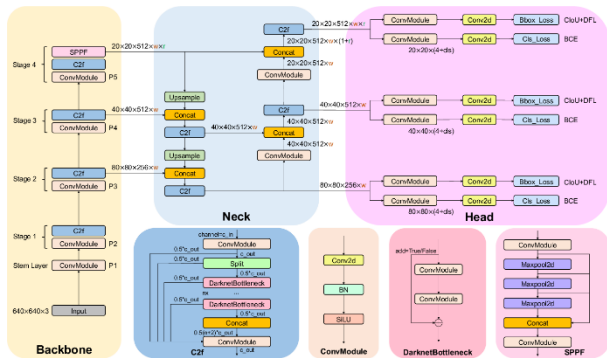
شکل ۲: معماری شبکه هشتم YOLO.
