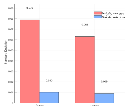
شکل ۵: کاهش انحراف معیار شاخص PSNDb پس از حذف رگبرگها
