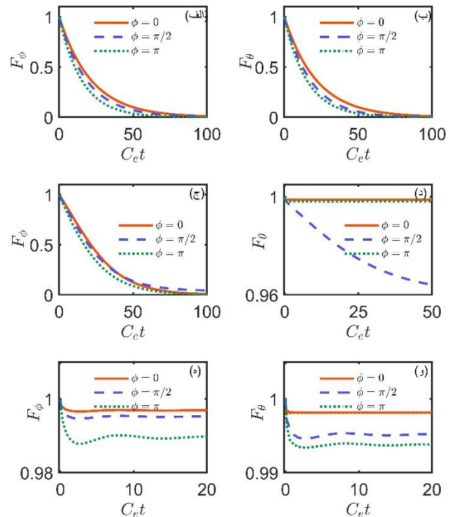
شکل ۲: دینامیک اطلاعات فیشری کوانتومی بر حسب تابعی از زمان مقیاس \theta = \frac{\pi}{2} و برای فازهای نسبی متفاوت با شرایط اولیه C_e t شده برای (ج) و (د) \Delta_a = -30c_e, \Delta_b = 10c_e برای (الف) و (ب)، \Delta_a = 10c_e, \Delta_b = 10c_e برای (ه) و (و). \Delta_a = -2c_e, \Delta_b = -10c_e
