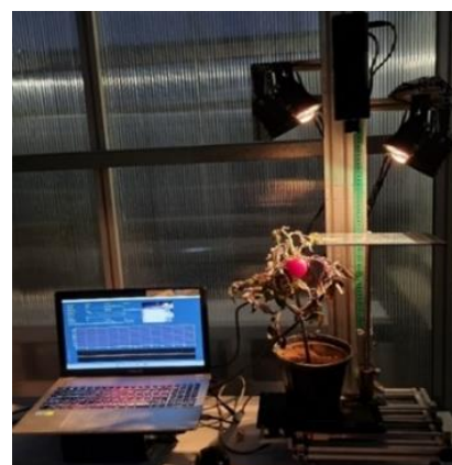
شکل ۱: چیدمان دوربین فراطیفی ونحوه داده‌گیری از برگ.
