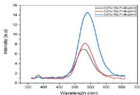
(ب) طیف فلورسانس CdTe در سه دمای مختلف ۳۰، ۶۰ و ۸۰ درجه سلیسیوس، زمان واکنش ۴ ساعت و pH=9
