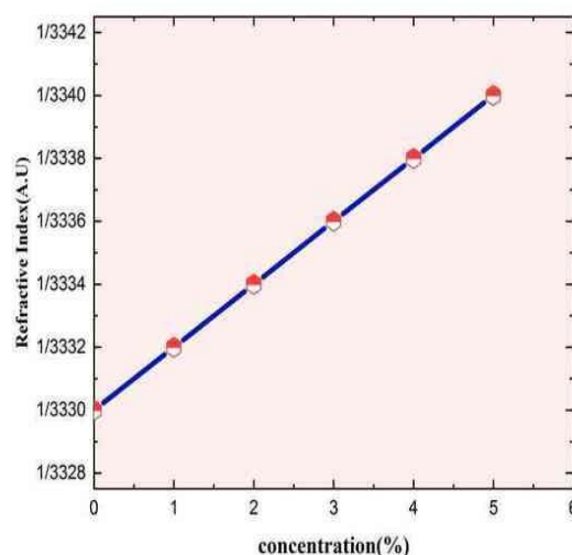
شکل ۴. نمودار تغییر ضریب شکست به ازای تغییر غلظت متانول محلول در آب از ۰ تا ۵٪
