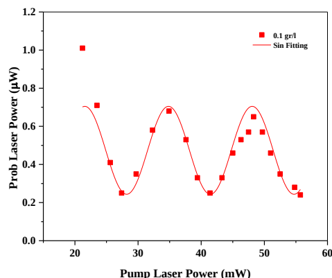
شکل ۴: تغییرات متناوب شدت حلقه‌های لیزر آزمون بر اساس لیزر پمپ
