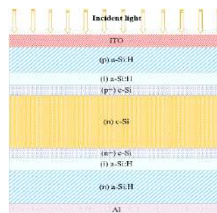
شکل ۲: شمای کلی سلول خورشیدی ناهمگون با لایه های بافر
