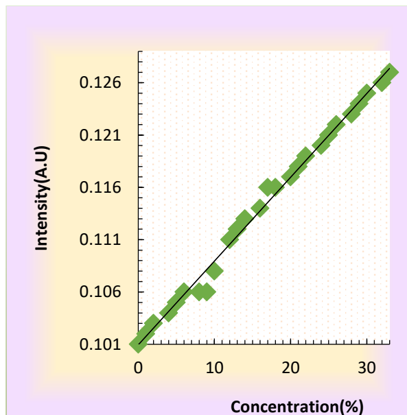
شکل ۲. نمودار تغییرات شدت نور بازتابی از ساختار تشدید پلاسمون سطحی برای غلظت‌های متفاوت متانول محلول در آب
