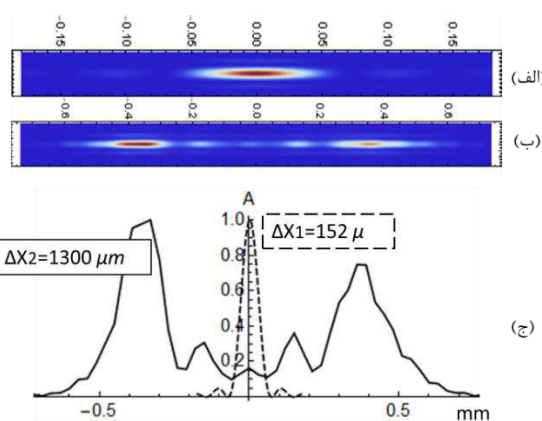
شکل ۵: شبیه سازی نمایه پراش باریکه لیزر عبوری از کریستال اینواسلب قبل (الف) و بعد (ب) از اعمال دمش با توان ۳۰۰ W. (ج) توزیع شدت به‌نچار شده لکه لیزر در دو حالت ذکر شده.
