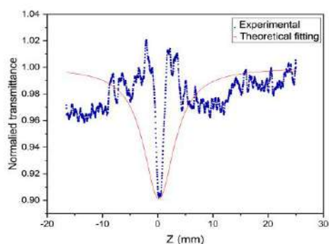
شکل ۲ (الف) نمودار میزان تراگسیل به ازای موقعیت مختلف نمونه در چیدمان روزنه باز در روش جاروب Z (الف) با استفاده از لیزر دیودی ماژول با طول موج ۵۳۲ نانومتر و توان لیزر ۳۲ میلی وات
