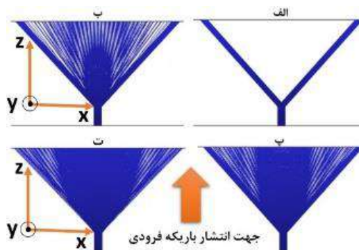
شکل ۴: انتشار پرتوها پس از عبور از عدسی خطی‌ساز برای شعاع انحنای مختلف نوک دندانه. الف: دندانه‌های کاملاً تیز، ب: ۰,۱ میلی‌متر، پ: ۰,۲ میلی‌متر و ت: ۰,۳ میلی‌متر
