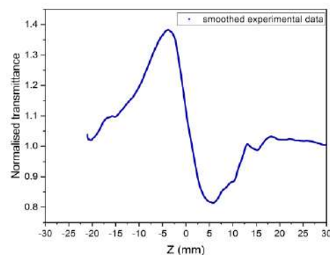
شکل ۳- نمودار میزان تراگسیل به ازای موقعیت مختلف نمونه در چیدمان روزنه بسته در روش جاروب Z الف) با استفاده از لیزر دیودی ماژول با طول موج ۵۳۲ نانومتر و توان لیزر ۳۲ میلی وات
