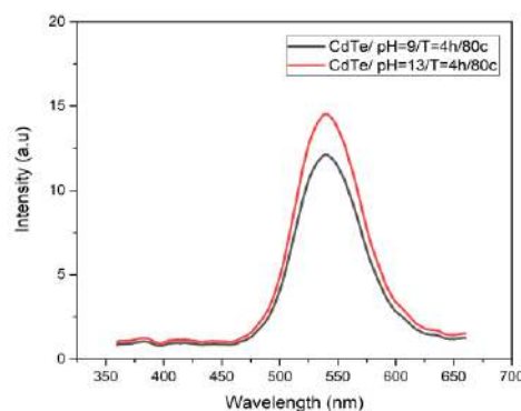
(ج) طیف فلورسانس CdTe در دو مقدار مختلف 9, 13 pH، زمان واکنش ۴ ساعت و دمای ۸۰ درجه سلیسیوس
