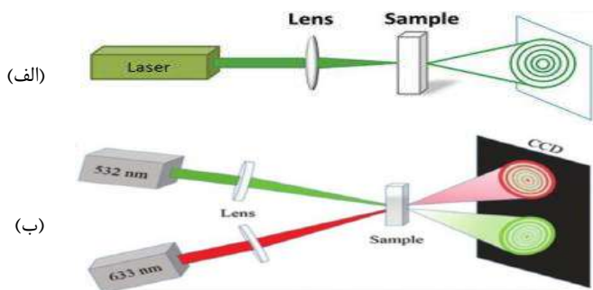
شکل ۱: چیدمان اپتیکی آزمایش (الف) SSPM و (ب) SXPM
