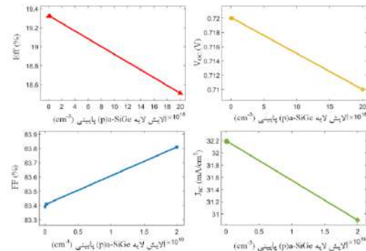
شکل ۵: کمیت‌های سلول طراحی‌شده به عنوان تابعی از غلظت آلایش لایه (p) a-SiGe پایینی (BF-(p) a-SiGe)
