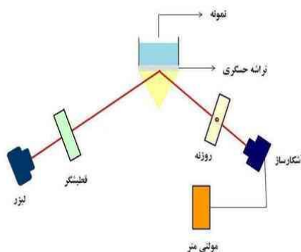
شکل ۱. چیدمان حسگری تشدید پلاسمون سطحی
