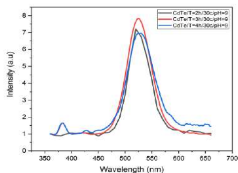
شکل ۱- (الف) طیف فلورسانس CdTe در سه بازه زمانی ۲ و ۳ و ۴ ساعت، دمای ۳۰ درجه و pH=9
