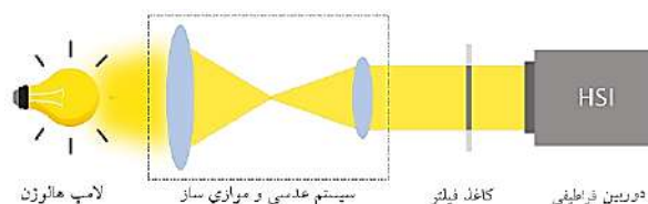
شکل ۲: شماتیکی از چیدمان تجربی آزمایش برای ثبت داده‌های فراطیفی لکه‌های غباری
