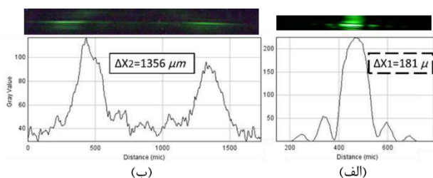
شکل ۶: (الف) تصاویر تجربی پراش باریکه لیزر عبوری از کریستال اینواسلب به‌همراه توزیع شدت آنها در دمش خاموش (ب) و روشن
