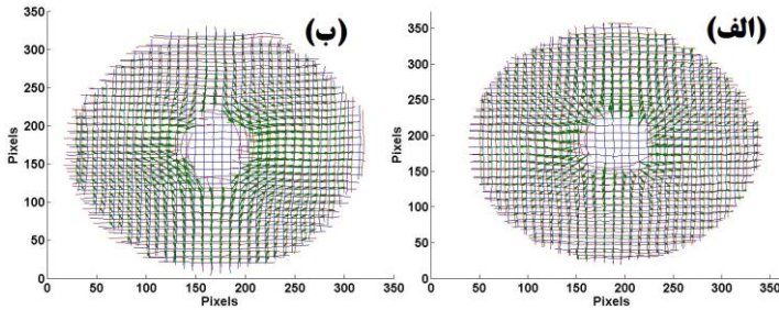
شکل ۵: الف: بردارهای جابه‌جایی الگوی ماره در آرایش شکل ۳- الف و ب: در آرایش شکل ۳- ب
