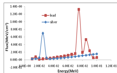
شکل ۸: مقایسه شار اشعه ایکس تولید شده برحسب انرژی برای هدفهای تیغه ای سرب و نقره با ضخامت ۲۰۰۰ میکرون.
