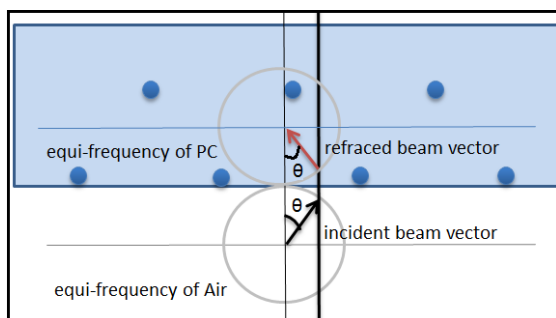
شکل ۳: نمودار کانتور هم‌فرکانس بلور فوتونی مثلثی و هوا در فرکانس \frac{0.222}{a} \frac{2\pi c}{a} . هر دو نمودار با هم یکسانند. زاویه ورودی و شکست \theta با هم برابر است.
