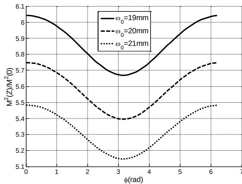
شکل ۱: تغییرات کیفیت پرتو نرمال شده برحسب تاخیر فاز ( \varphi ) برای کمره پرتوهای مختلف در اتمسفر متلاطم.
