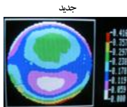
شکل ۱۹، نمایش ناهمواری جبهه موج در نتیجه عبور از سله، پس
