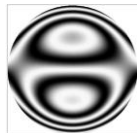
شکل ۴، الگوی تداخلی حاصل از جابه‌جا شدن عدسی ۲، به میزان DCY=0.1mm
