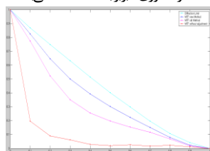
شکل ۲۰، مقایسه منحنی MTF در سله های که به روش جدید تنظیم شده است، با منحنی
