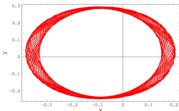
شکل ۱: نمودار مقطع عرضی مسیر حرکت تک ذره در ویگلر لیزری برای \Omega_0 = 0.42 و \Omega_L = 0.05 ، \gamma = 8 .
