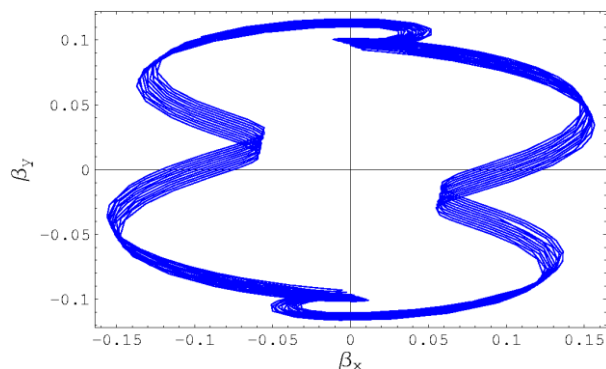
شکل ۲: نمودار برش عرضی سرعت های بهنجار (\beta_x, \beta_y) برای \Omega_0 = 0.38 و \Omega_L = 0.05 ، \gamma = 8 .
