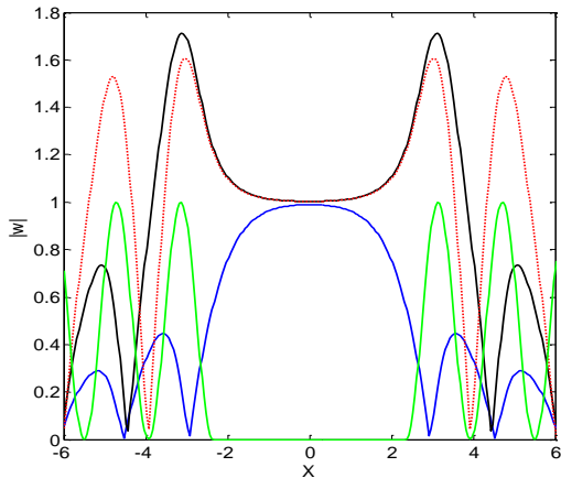
شکل ۴: مقایسه پروفایل مد تک قطبی (خط آبی)، دوسطی نوع I (خط مشکی) و دوسطی نوع II (نقطه چین قرمز) در اطراف هسته مرکزی. خطوط متناوب سبز تابع مدولاسیون ضریب شکست R(x) را نشان می‌دهند.
