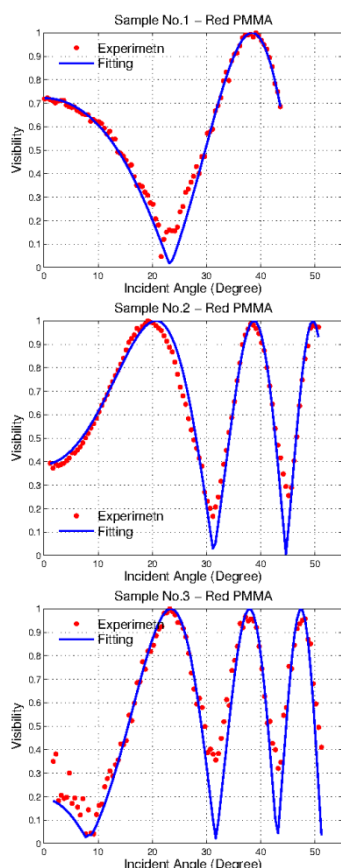
شکل ۴: منحنی نمایانی بر حسب زاویه فرود. نقاط، نشان دهنده داده‌های تجربی (پس از حذف نمودن نوفه‌های زمینه) و خط ممتد، بهترین نمودار نظری برازش شده است.
