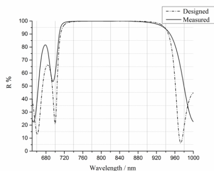
شکل ۴: منحنی‌های بازتابندگی طراحی شده و اندازه‌گیری شده.
