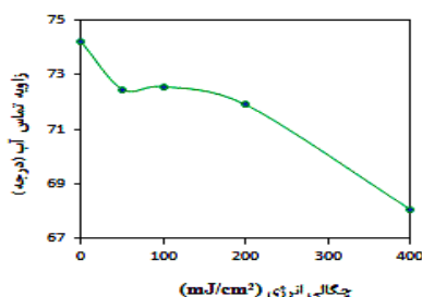
شکل ۷: نمودار تغییر زاویه تماس آب با سطح پلیمر PADC بر حسب شاریدگی در تابش‌دهی با ۲۵۰ تپ.
