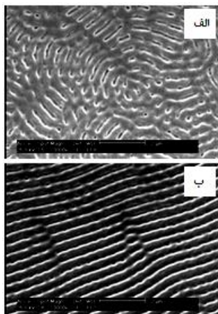
شکل ۴: تصویر SEM برای پلیمر PADC تابش‌دهی شده با لیزر ArF با شاریدگی 500 \text{ mJ/cm}^2 (الف) و 50 تپ و 1000 تپ.
