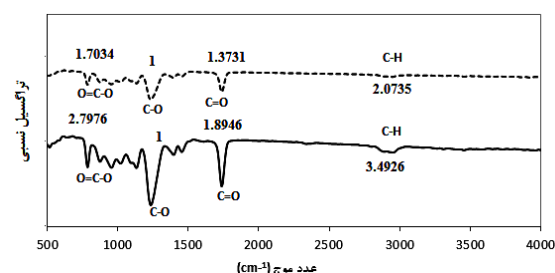
شکل ۶: شدت بهنجار شده برای طیف فروسرخ PADC خام (خط پر) و پلیمر تابش‌دهی شده با لیزر ArF با شاریدگی ۵۰۰ mJ/cm ۲ و با ۱۰۰۰ تپ (خط‌چین).
