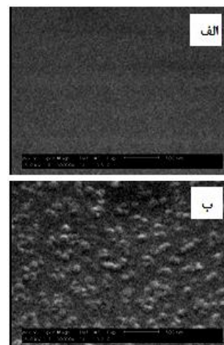
شکل ۳: تصویر SEM پلیمر PADC تابش‌دهی شده با لیزر ArF با شاریدگی 50 \text{ mJ/cm}^2 (الف) و 300 تپ و 3000 تپ.
