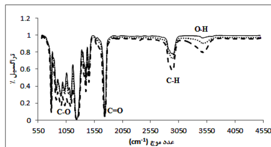
شکل ۵: طیف فروسرخ برای PADC خام (خط پیوسته) و پلیمر تابش‌دهی شده با لیزر ArF با شاریدگی ۵۰ mJ/cm ۲ و با ۳۰۰ تپ (نقطه‌چین) و ۳۰۰۰ پالس (خط‌چین).
