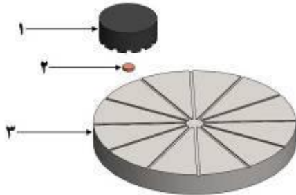
شکل ۱: ترتیب قرار گیری اجزای فرآیند بر روی صفحه پولیش میانی. نواحی ۱، ۲ و ۳ به ترتیب عبارتند از: وزنه استیل، قرص مس، صفحه پولیش میانی
