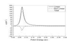
شکل ۳: تغییرات ضریب جذب خطی، غیرخطی مرتبه سوم و کل براساس انرژی
