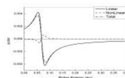
شکل ۲: تغییرات ضریب شکست خطی، غیرخطی مرتبه سوم و کل به ازای R = 42A^0 , w = 20A^0 , B = 10T فوتون، انرژی، فوتون، و
