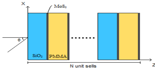
شکل ۱: ساختار بلور فوتونی یک بعدی حاوی مولبدین دی سولفاید.
