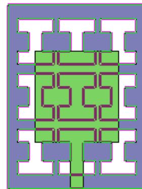
شکل ۳: آنتن مایکرواستریپ بلور فوتونی
