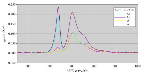
شکل ۲: طیف تحریک و گسیل متیلن‌بلو در گلیسرین (طول موج تحریک ۶۳۰nm) بازای زوایای افقی و عمودی قطبشگر و تحلیلگر
