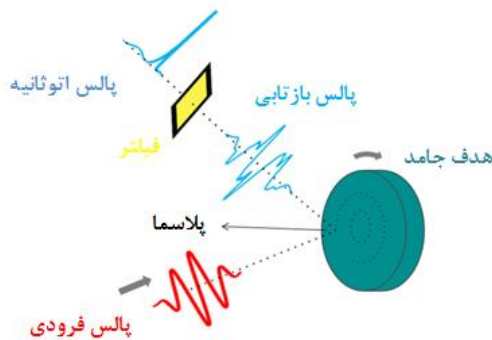
شکل ۱ طرحواره برهمکنش لیزر با پلاسما و تولید هارمونیکهای بالا و تولید پالس اتوثانیه
