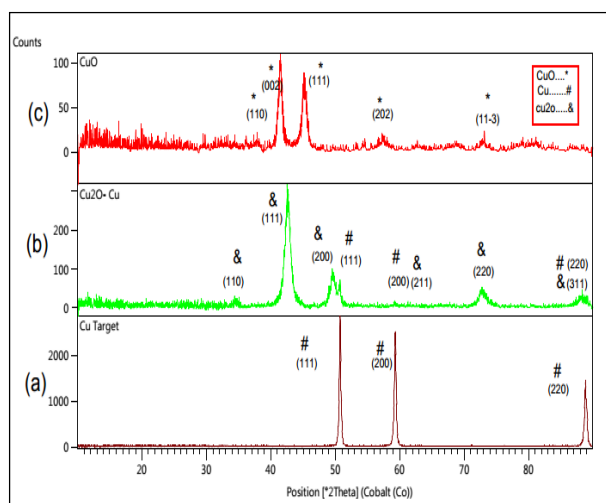
شکل ۳: طیف پراش اشعه X (a) ورقه مس خالص (b) نانوذرات CuO و (c) نانوذرات CuO ساخته شده، با لیزر تپی
