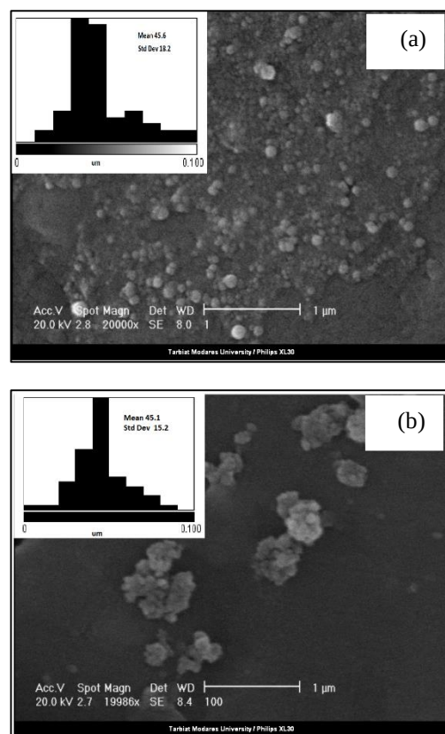
شکل ۴: تصاویر SEM و توزیع نانوذرات مربوط به (a) Cu/Cu 2 O و (b) نانوذرات CuO
