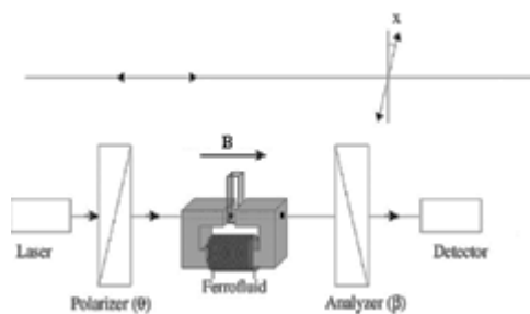
شکل ۱: چیدمان فارادی.
