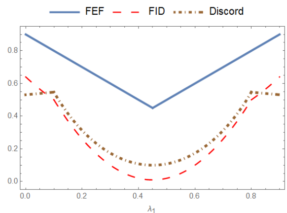
شکل ۳: نمودار کمیت‌ها برحسب \lambda_1 به ازای \lambda_3 = 0.1 ، \lambda_4 = 0 و \lambda_2 = 1 - \lambda_1 - \lambda_3 - \lambda_4 .
