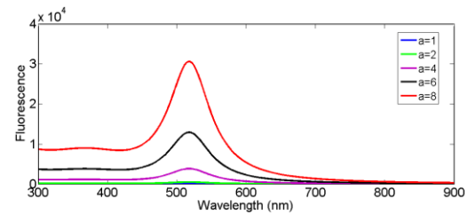
شکل (۲): طیف گسیلی فلورسانس نانوذرات کروی با در نظر گرفتن مدل درود
