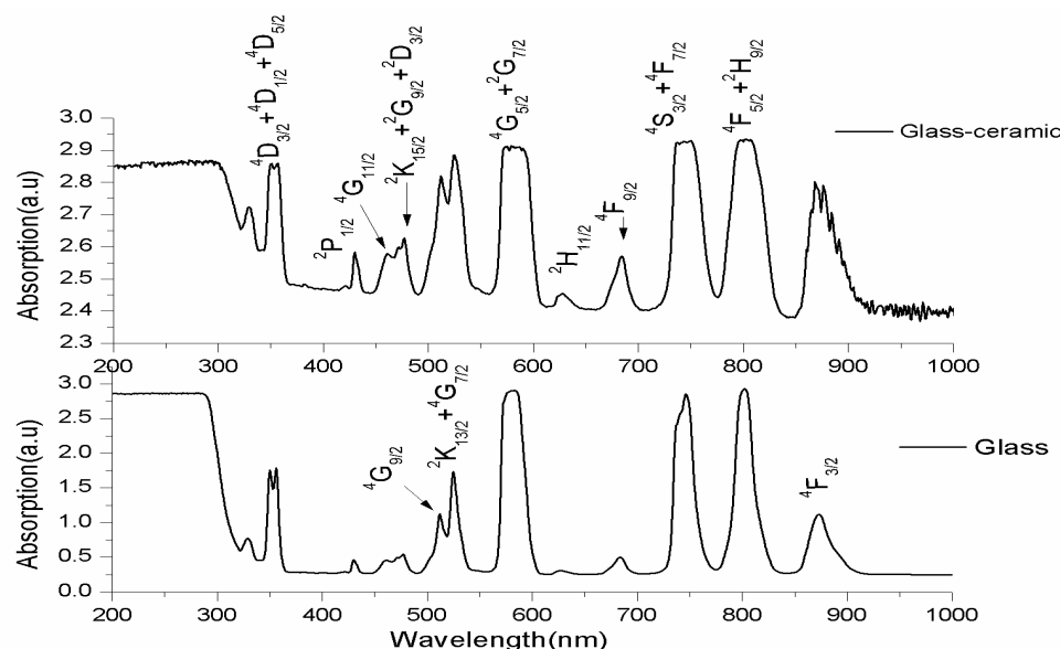
شکل ۱: طیف جذبی نمونه شیشه و شیشه-سرامیکی آلاینده به \text{Nd}^{3+} در بازه ۲۰۰-۱۰۰۰ nm در دمای اتاق، همه گذارها از تراز 4I_{9/2} می‌باشد و گذار مربوط به هر قله بر روی آن مشخص شده است.
