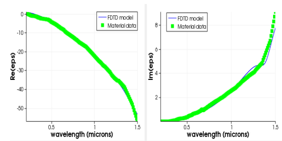
شکل ۲: قسمت حقیقی و موهومی ثابت دی الکتریک \epsilon_2(\omega) بر حسب طول موج [۲].
