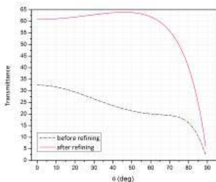
شکل ۲- منحنی تراگسیل قبل و بعد از بهینه سازی سامانه پنج لایه ای برحسب محدوده ی زاویه ی تابش نور فرودی با طول موج (nm) ۵۰۰
