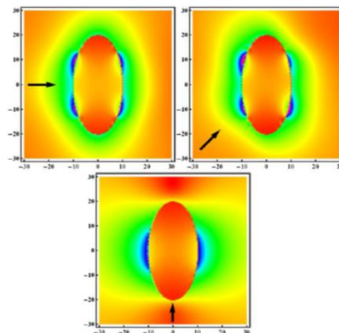
شکل ۴) توزیع اندازه میدان الکتریکی در مقطع نانوسیم بیضوی با زاویه تابش‌های صفر، ۴۵ و ۹۰ درجه (محورها بر حسب نانومتر هستند).
