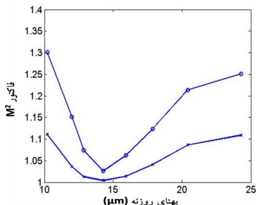
شکل ۶: ضریب M^2 در راستای x برای پهنای متفاوت روزنه محدودکننده میدان در تشدیدگر SFUR. نماد (\times) تشدیدگر با حضور بهره و (O) نماد تشدیدگر بدون حضور بهره است.
