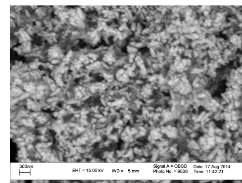
شکل ۳-ج: تصویر SEM اکسید کادمیم ۱٪ آلاینده شده با آهن
