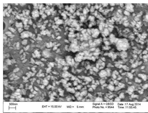
شکل ۳-ب: تصویر SEM اکسید کادمیم ۰/۵٪ آلاینده شده با آهن
