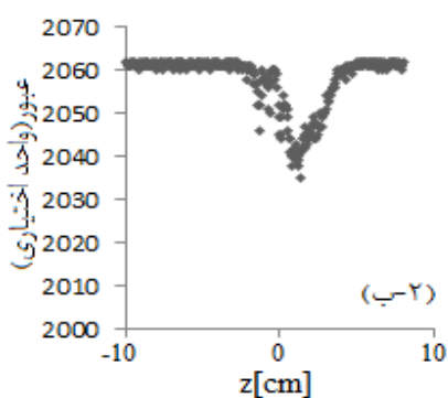
شکل-۲: (الف): نمودار عبور از روزنه بسته بصورت تابعی از z برای شکست غیرخطی قبل از تابش \beta . (ب): نمودار عبور از روزنه باز بصورت تابعی از z برای جذب غیرخطی قبل از تابش \beta .
