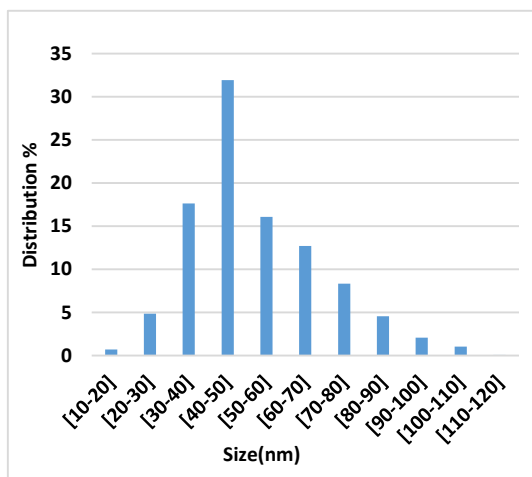
شکل ۱: نمودار توزیع اندازه نانوذرات TiO_2 .
