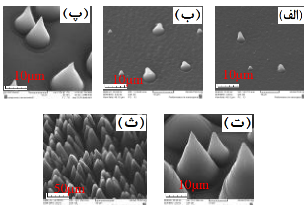
شکل ۲: نمونه‌های PET تابش‌دهی شده با شاریدگی 100 \text{ mJ/cm}^2 و تعداد تپ (الف) ۵۰، (ب) ۱۰۰، (پ) ۲۵۰، (ت) ۵۰۰، (ث) ۱۰۰۰.
