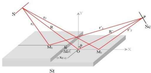
شکل ۱: شمای پراش فرنل از لبه فازی. S چشمه خطی به موازات لبه پله St ، پله و Sc پرده مشاهده عمود بر باریکه بازتابیده است.
