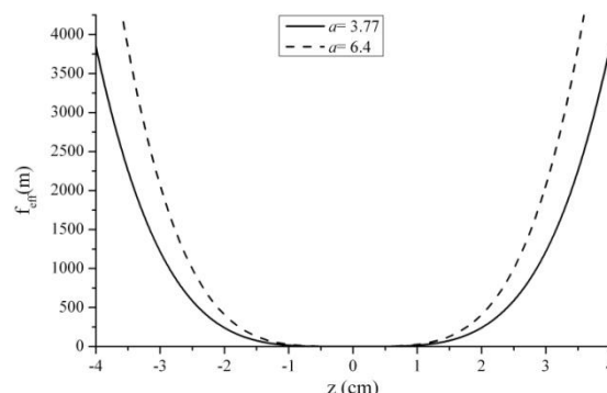
شکل ۴: تغییرات فاصله کانونی مؤثر ماده غیرخطی برحسب فاصله از محل کمر باریکه لیزری. فاصله‌های کانونی برای دو مقدار حدی ضریب اصلاحی a در رابطه (۱۰) رسم شده‌اند. افت شدید قدرت کانونی کندگی عدسی؛ با دور شدن از محل کمر باریکه مشهود است.
