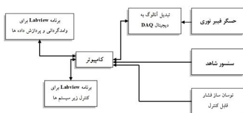
شکل ۲: نمایش شماتیک از اجزای مختلف سخت افزای و نرم افزاری حسگر.
