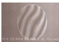
شکل ۱۶: الگوی تداخلی حاصل از آزمون MTF بر روی سامانه‌ی تصویربرداری پس از انجام تنظیمات
