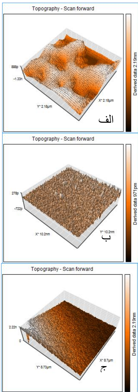
شکل ۱: تصویر AFM فیلم های پلیمری ایجاد شده تحت شرایط مختلف. الف) خلا و نور فرابنفش ب) پلاسمای هلیوم ج) میدان الکتریکی و نور فرابنفش
