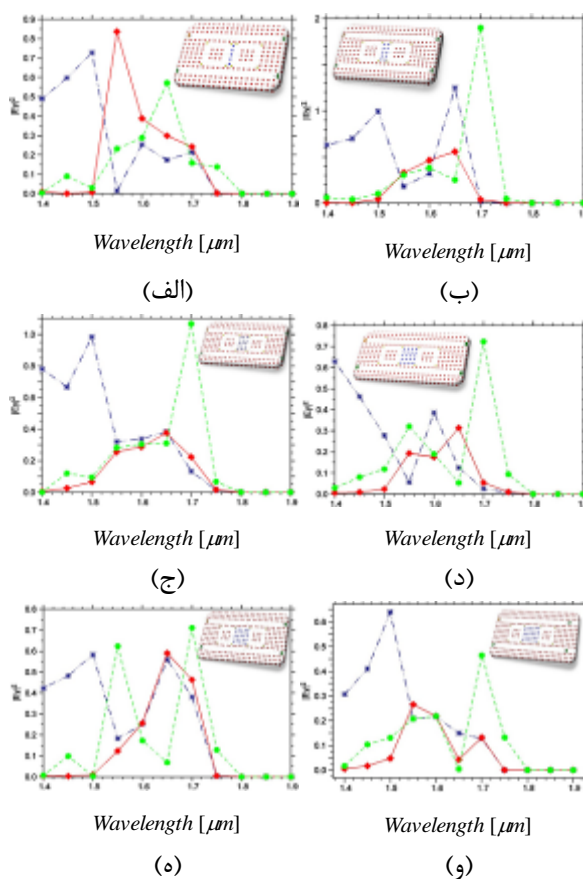
شکل ۴: پاسخ طیفی توان انتقالی ساختار تشدیدگر حلقوی دوتایی بلور فوتونی در هندسه موازی، نمودار خط‌پر (کانال C)، خط تیره (کانال D) و خط تیره - دو نقطه (کانال B)
