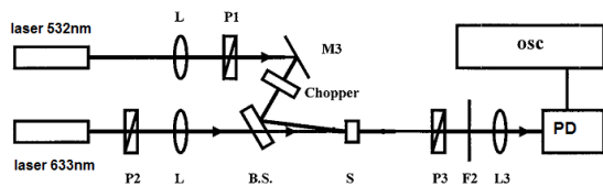
شکل ۱: چیدمان دوشکستی القایی: P 1 : پلاریزور، L s : لنز، M 3 : آینه، S: نمونه، F 2 : فیلترسبز، PD: آشکارساز، OSC: اسیلوسکوپ، B.S.: شکافنده پرتو.
