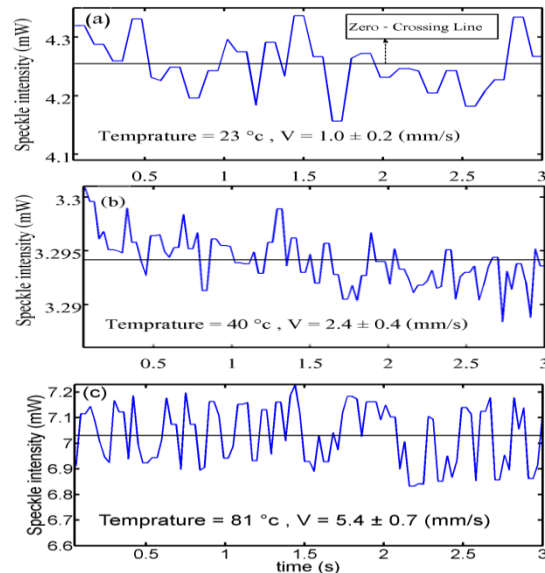
شکل ۳: نمودار توان بر حسب زمان برای دماهای مختلف نمونه
