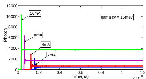
شکل ۶: تحولات زمانی فوتونها در جریانهای تزریقی ۲، ۴، ۸ و ۱۶ میلی آمپر و در پهن شدن همگن با FWHM، ۱۵ meV
