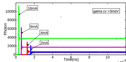
شکل ۵: تحولات زمانی فوتونها در جریانهای تزریقی ۲، ۴، ۸ و ۱۶ میلی آمپر و در پهن شدن همگن با FWHM، ۳ meV
