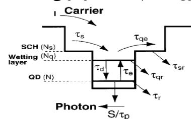
شکل ۱: نمای نوار رسانش در منطقه فعال لیزر و مراحل واهلش حاملها به حالت پایه نقطه کوانتومی [۶]
