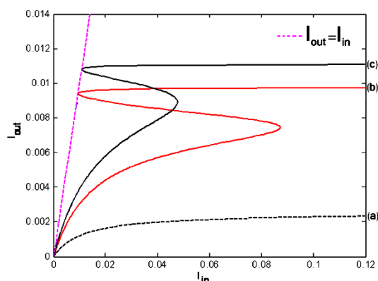
شکل ۲: اثر تعداد لایه های نقص در تراگسیل (a) بدون لایه نقص (b) با پنج لایه نقص (c) با شش لایه نقص.
