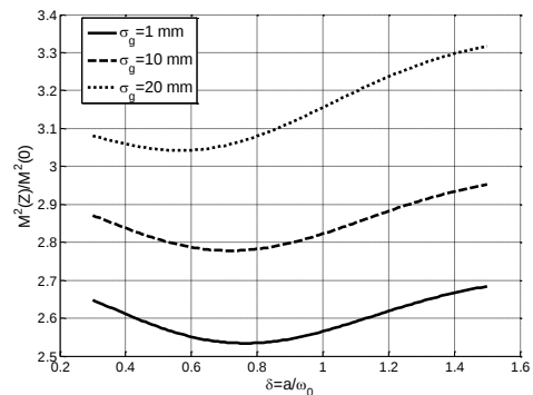
شکل ۴: تغییرات کیفیت پرتو بر حسب شعاعهای مختلف روزنه برای درجه همدوسی های مختلف منبع
