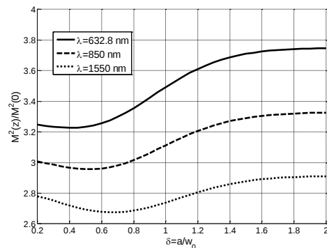
شکل ۵: تغییرات کیفیت پرتو بر حسب شعاعهای مختلف روزنه برای طول موجهای مختلف
