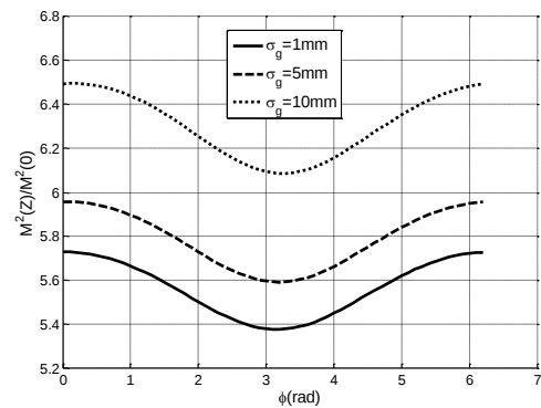
شکل ۳: تغییرات کیفیت پرتو نرمال شده بر حسب تاخیر فاز (\varphi) برای درجه همدوسی های مختلف منبع در اتمسفر متلاطم.
