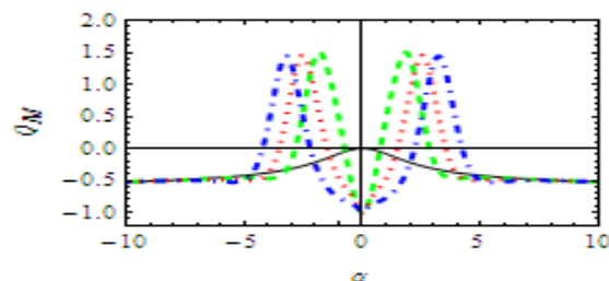
شکل ۱: پارامتر مندل برحسب مقادیر مختلف \alpha برای k = 0.0 ، n = 0, 3, 6, 10 (خط پیوسته، خط چین، نقطه چین، نقطه چین). به ازای مقادیر مختلف n ؛ n = 0 (خط پیوسته)، n = 3 (خط چین)، n = 6 (نقطه چین)، n = 10 (خط نقطه چین).
