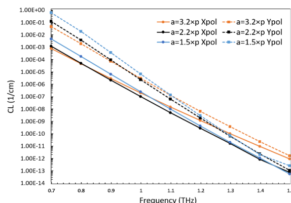
شکل ۴: تلفات تحدید برحسب فرکانس برای مدهای قطبشی X و Y در قطر های اصلی متفاوت از هسته
