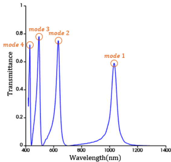
شکل ۲. طیف عبور ساختار پیشنهادی و نمایش مدهای مختلف تشدید در طول موج های 429nm، 494nm، 632nm، 1030nm و 1500nm
