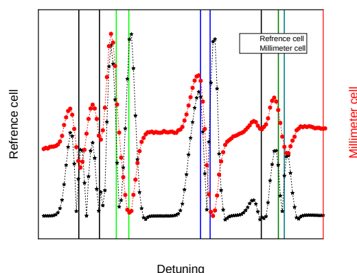
شکل ۴. داده اندازه گیری با مدولاسیون فرکانسی از سلول مرجع (ستاره و مشکی) و سلول میلیمتری (دایره و قرمز).
