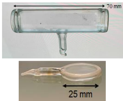
شکل ۱: از بالا سلول مرجع با ابعاد 70 \times 25 ، و سلول میلیمتری با ابعاد 3 \times 20 میلی‌متر.
