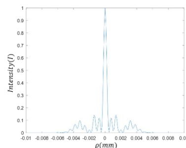
شکل ۳: شبیه‌سازی تحول میدان دور به ازای مقدار بیشینه تغییر فاز R=1.33 \text{ m} و \Delta\phi_0(z_0) = 8\pi .
