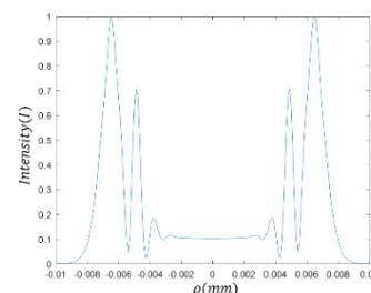
شکل ۴: شبیه‌سازی تحول میدان دور به ازای مقدار بیشینه تغییر فاز R=1.33 \text{ m} و \Delta\phi_0(z_0) = -8\pi .
