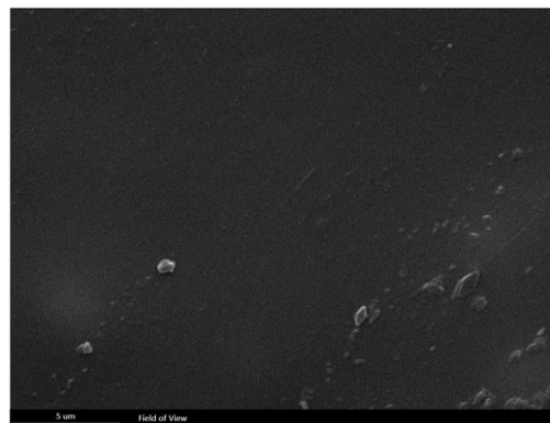
شکل ۴- تصویر SEM سطح سلول خورشیدی پروسکایتی کپسول شده با پلیمر پلی‌متیل‌متاکریلات
