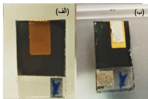
شکل ۴- تصویر سلول خورشیدی پروسکایتی قبل و بعد از لایه نشانی با لایه کپسول کننده پلی متیل متاکریلات
