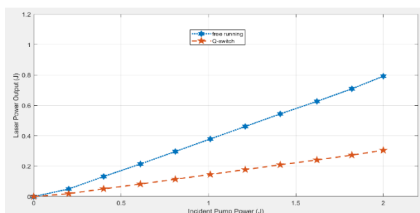
شکل ۳: انرژی نوری خروجی نوسانگر برحسب انرژی نوری دمشی مختلف
