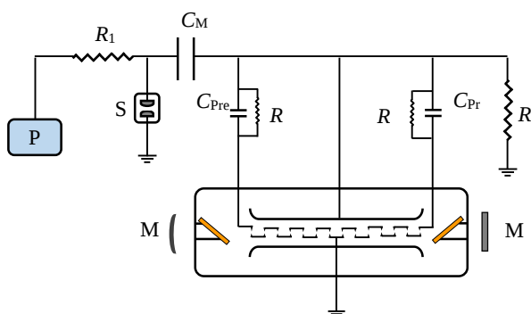
شکل ۱ شماتیک از لیزر \text{CO}_2 چند اتمسفری استفاده شده.
